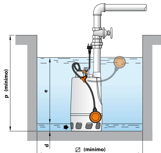
Instalación típica
